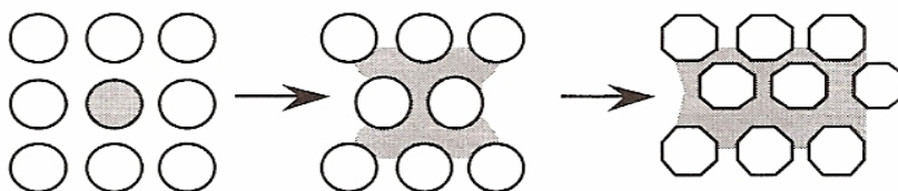
Slika 11. Mokro sinteriranje [4]
