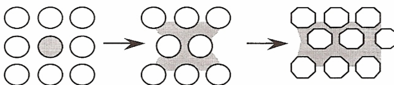
Slika 11. Mokro sinteriranje [4]
