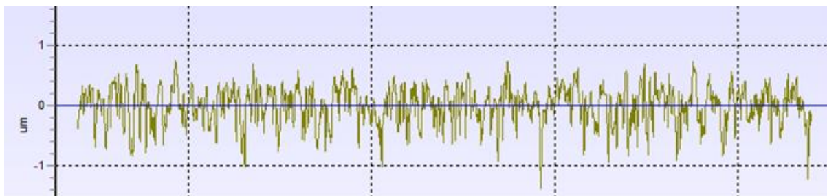
Slika 38. Profil hrapavosti osnovnog materijala za uzorak 2
