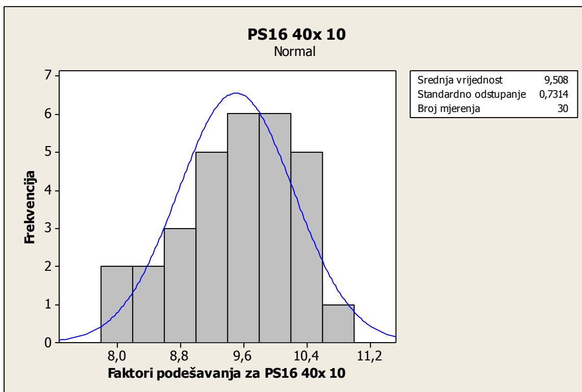
Slika 6.4. Histogram podešavanja mjernom skalom PS16 za povećanje 40x i duljinom podešavanja 10 μm
