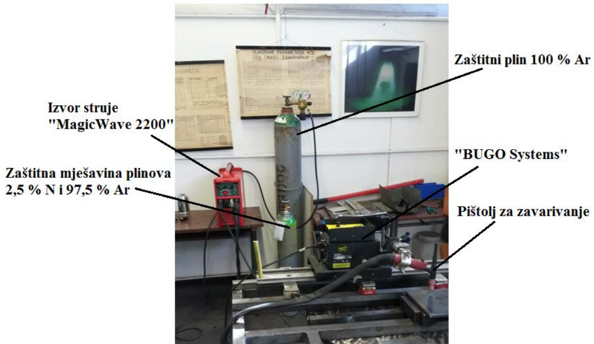
Slika 50. Radno mjesto u Laboratoriju za zavarivanje
