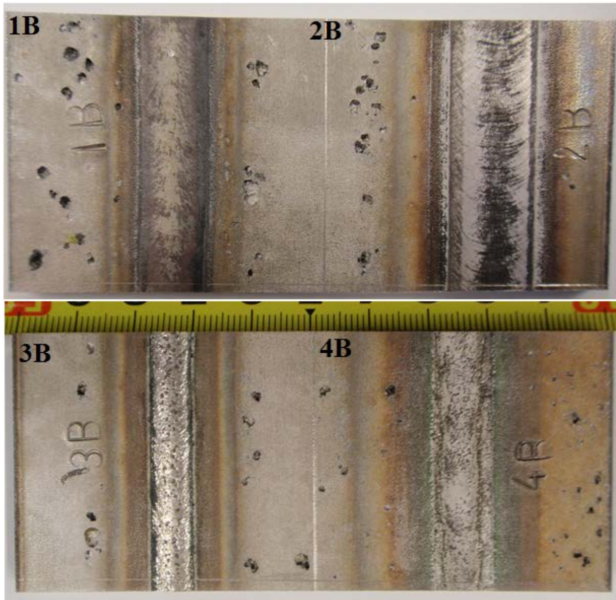
Slika 73. Izgled navarenih uzoraka (1B, 2B, 3B, 4B) nakon 48-satnog izlaganja agresivnoj otopini
