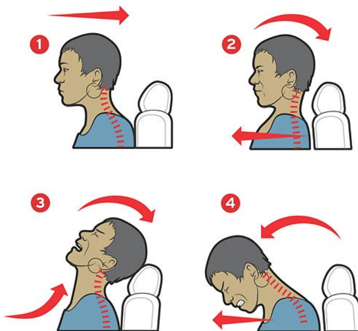
Slika 25. Faze whiplasha [14]
