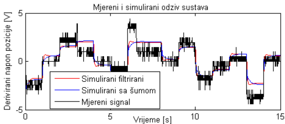
Slika 45. Mjereni i simulirani odziv sustava - PRMS (brzina)
