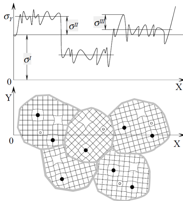
Slika 9. Prvi, drugi i treći red zaostalih napreznaja [5]
