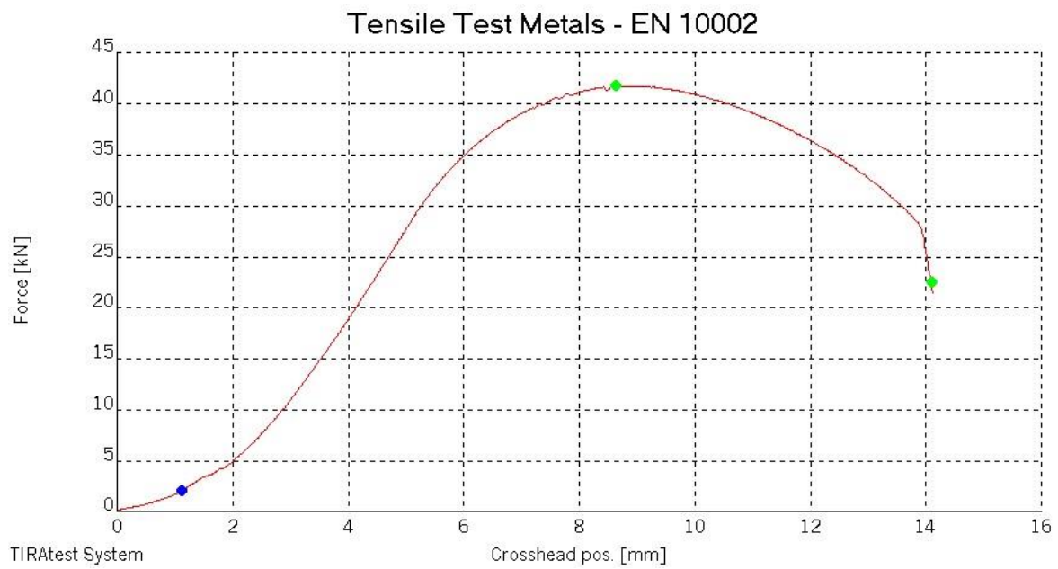
Slika 38. Graf sila-istezanje uzorak 2-1
