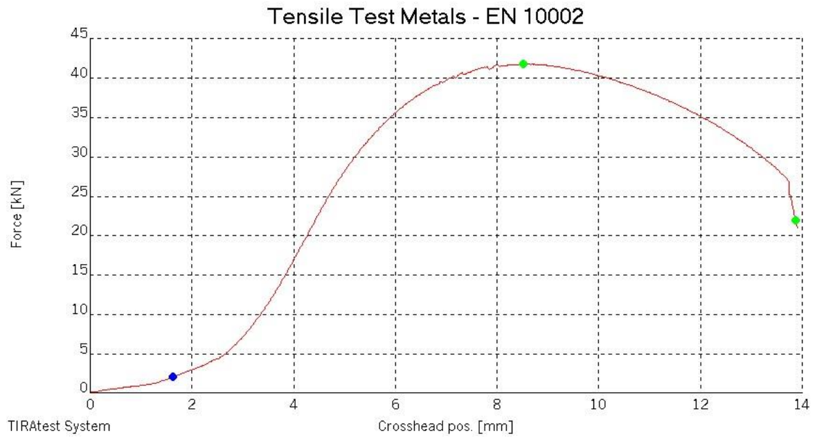
Slika 37. Graf sila-istezanje uzorak 1-1
