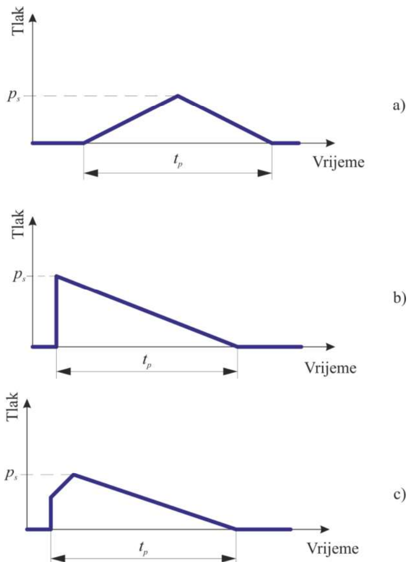
Slika 1.5. Pojednostavljeni dijagrami karakteristike eksplozije: a) brzo sagorijevanje, b) detonacija, c) kombinirano
