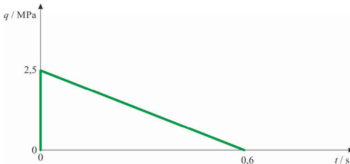
Slika 2.9. Dijagram opterećenja
