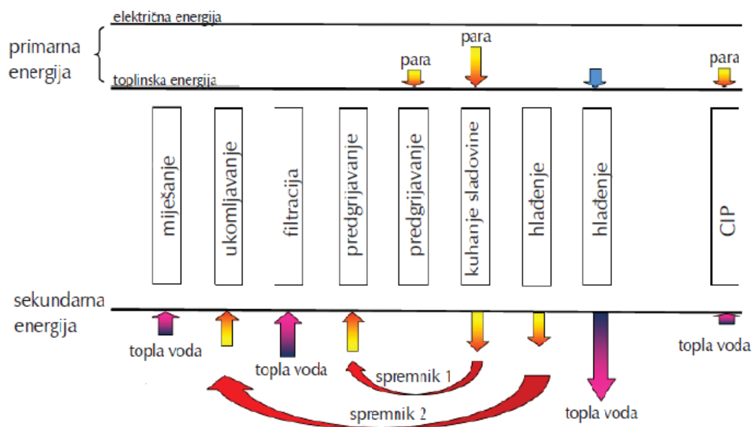
Slika 2. Toplina u procesu ukomlјavanja[4]
