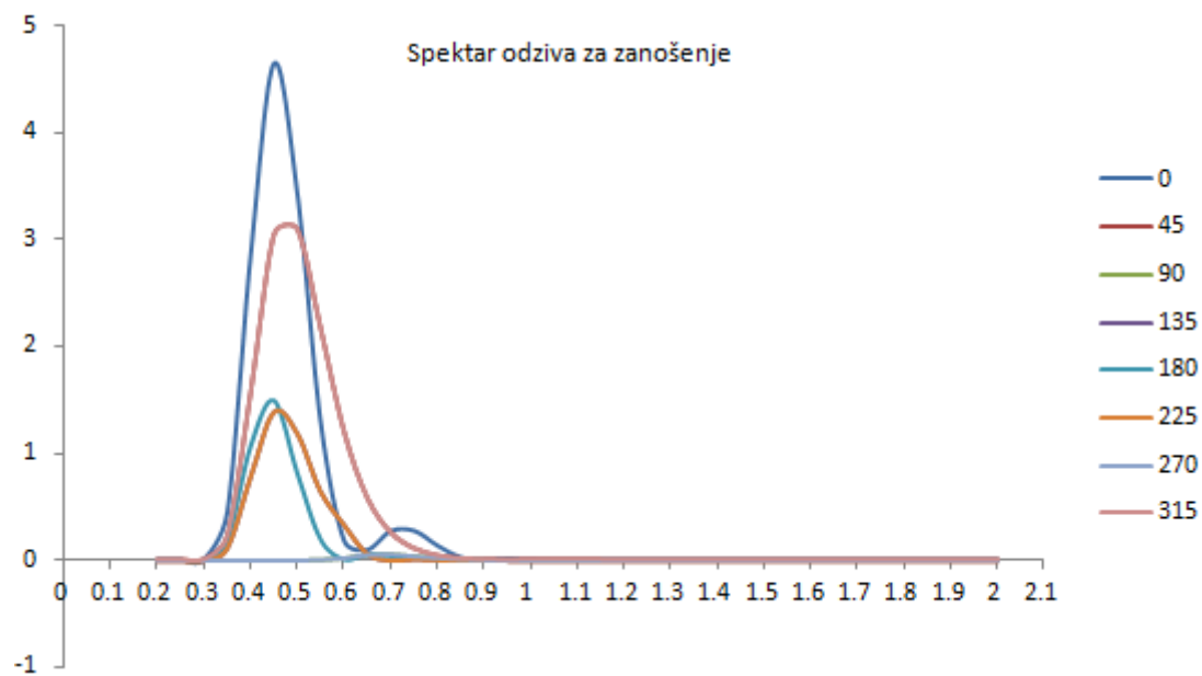
Slika 9. Spektar odziva za zanošenje, H_{1/3} = 7.20\text{m}
