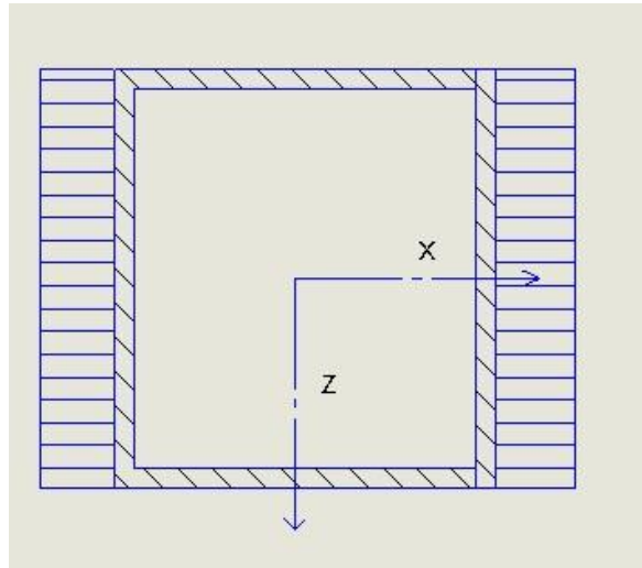
Slika 23 skica raspodjele smičnog naprežanja uslijed djelovanja sile
