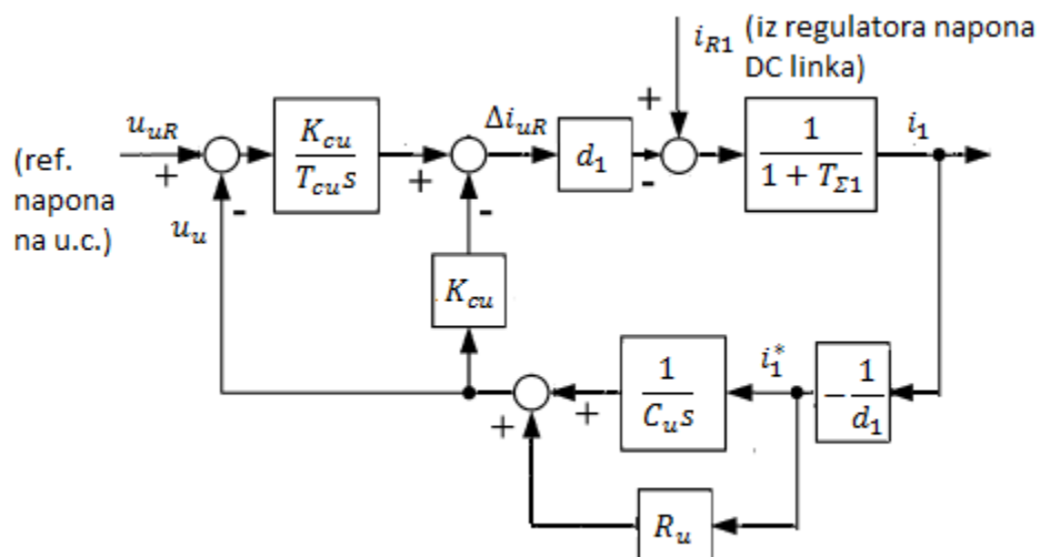
Slika 33 Struktura regulacijskog kruga SoC regulatora ultrakondenzatora
