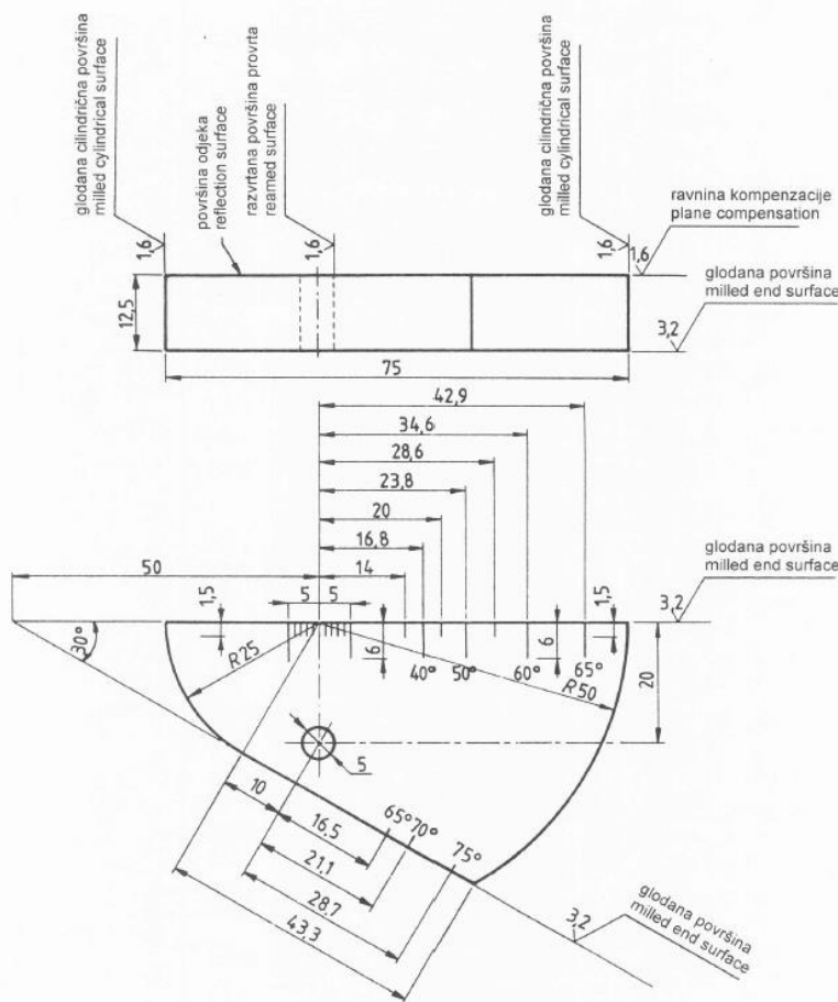
Slika 9. Dimenzije radnog etalona br.2 [8]
