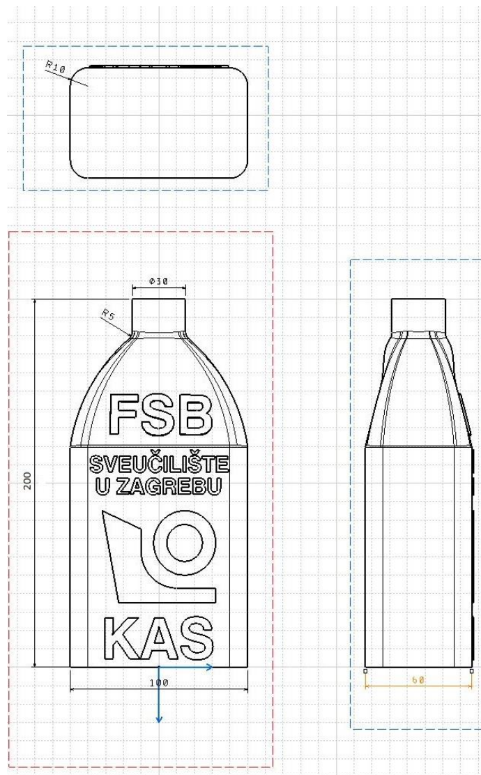
Slika 25. Dimenzije boce [7]
