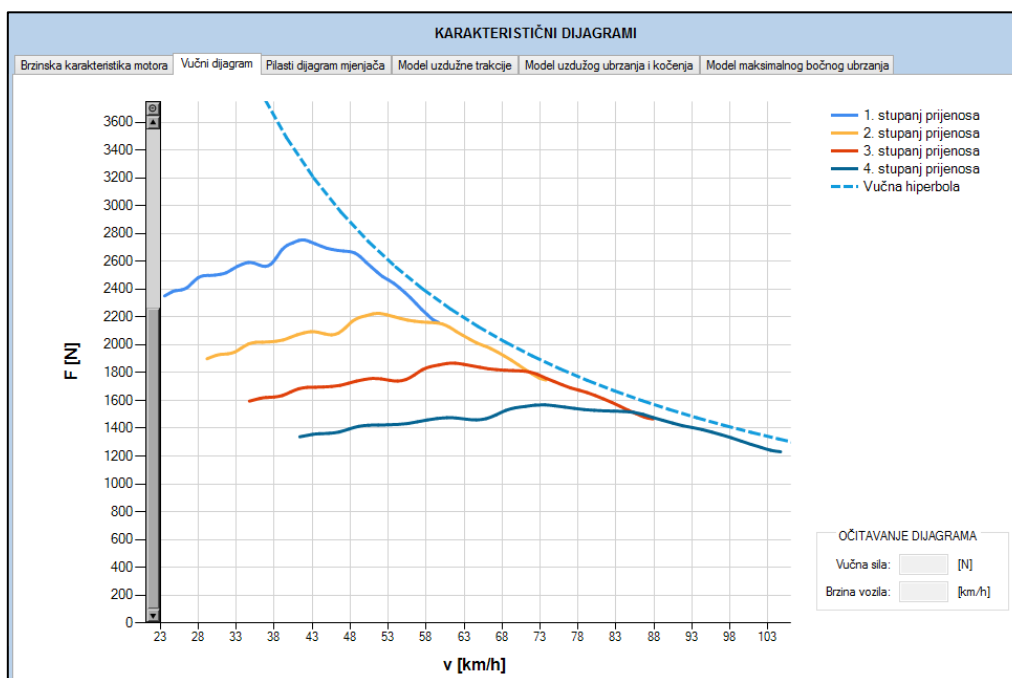
Slika 9. Vučni dijagram vozila Strix
