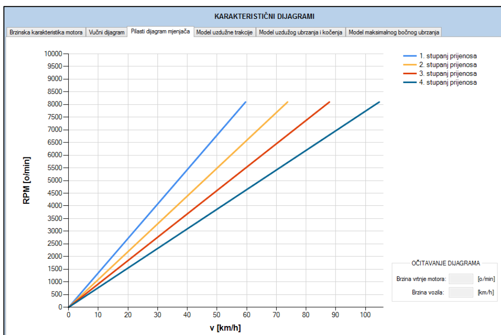
Slika 10. Pilasti dijagram mjenjača vozila Strix
