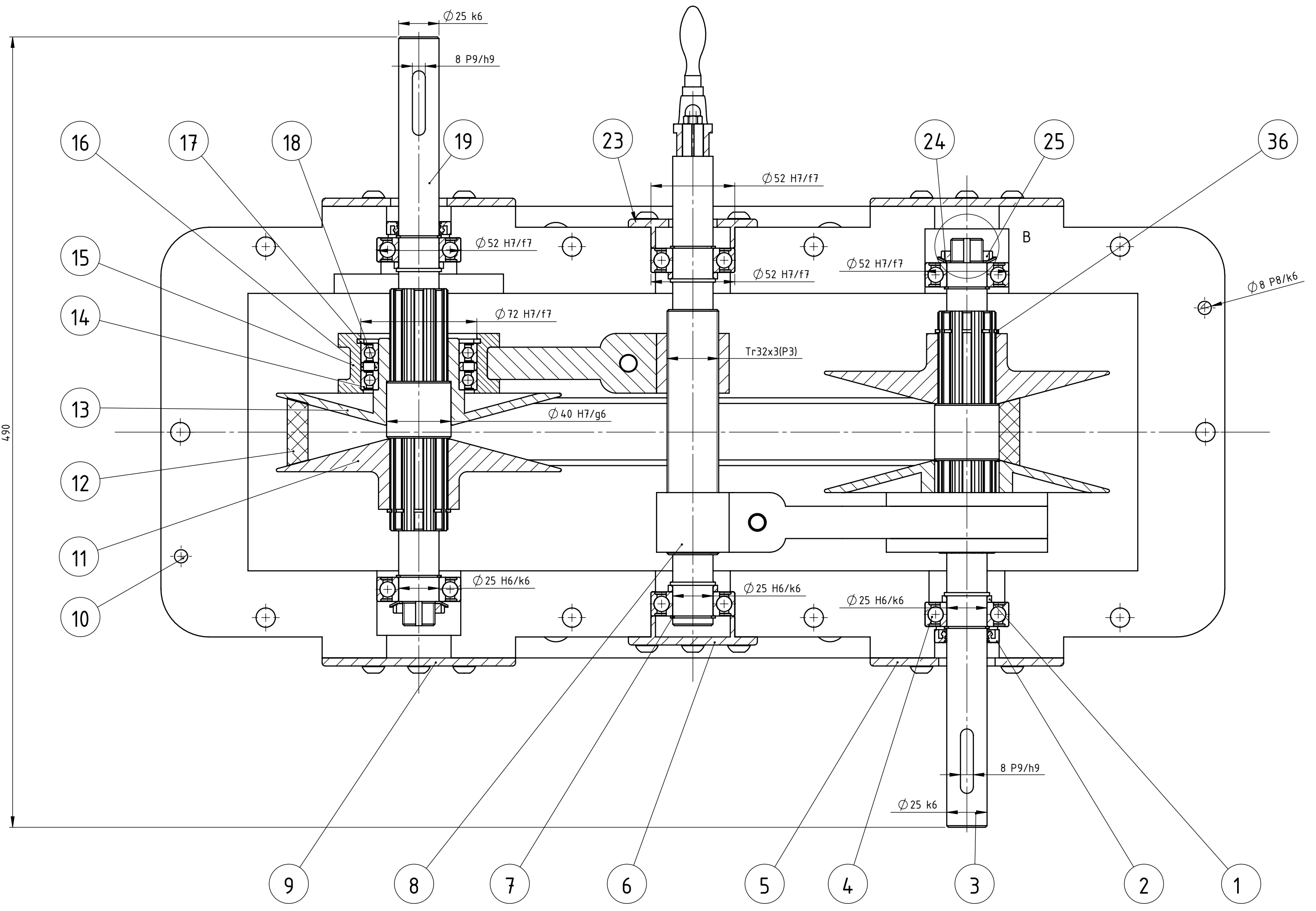
A-A (M 1:2)
