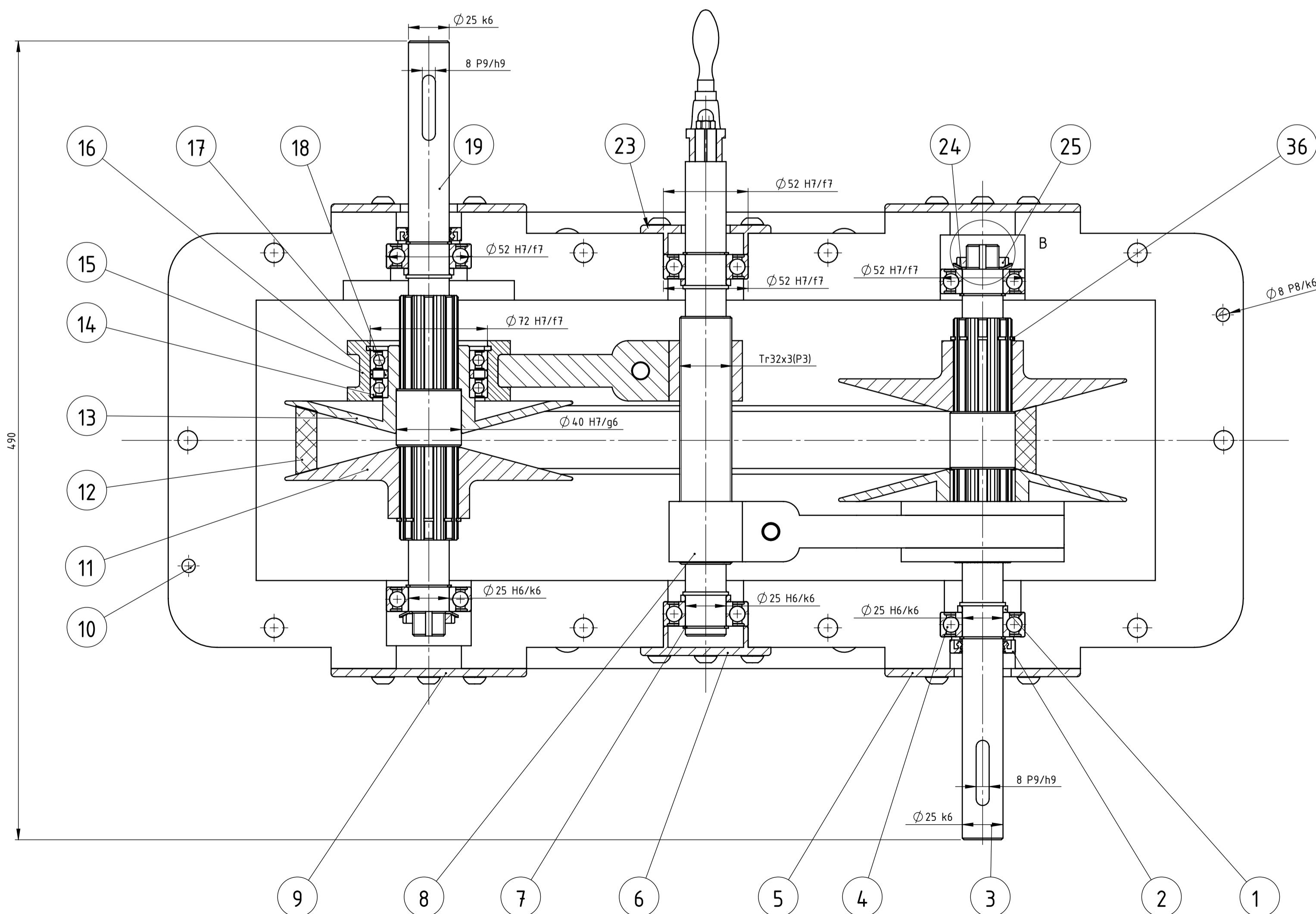
A-A (M 1:2)
