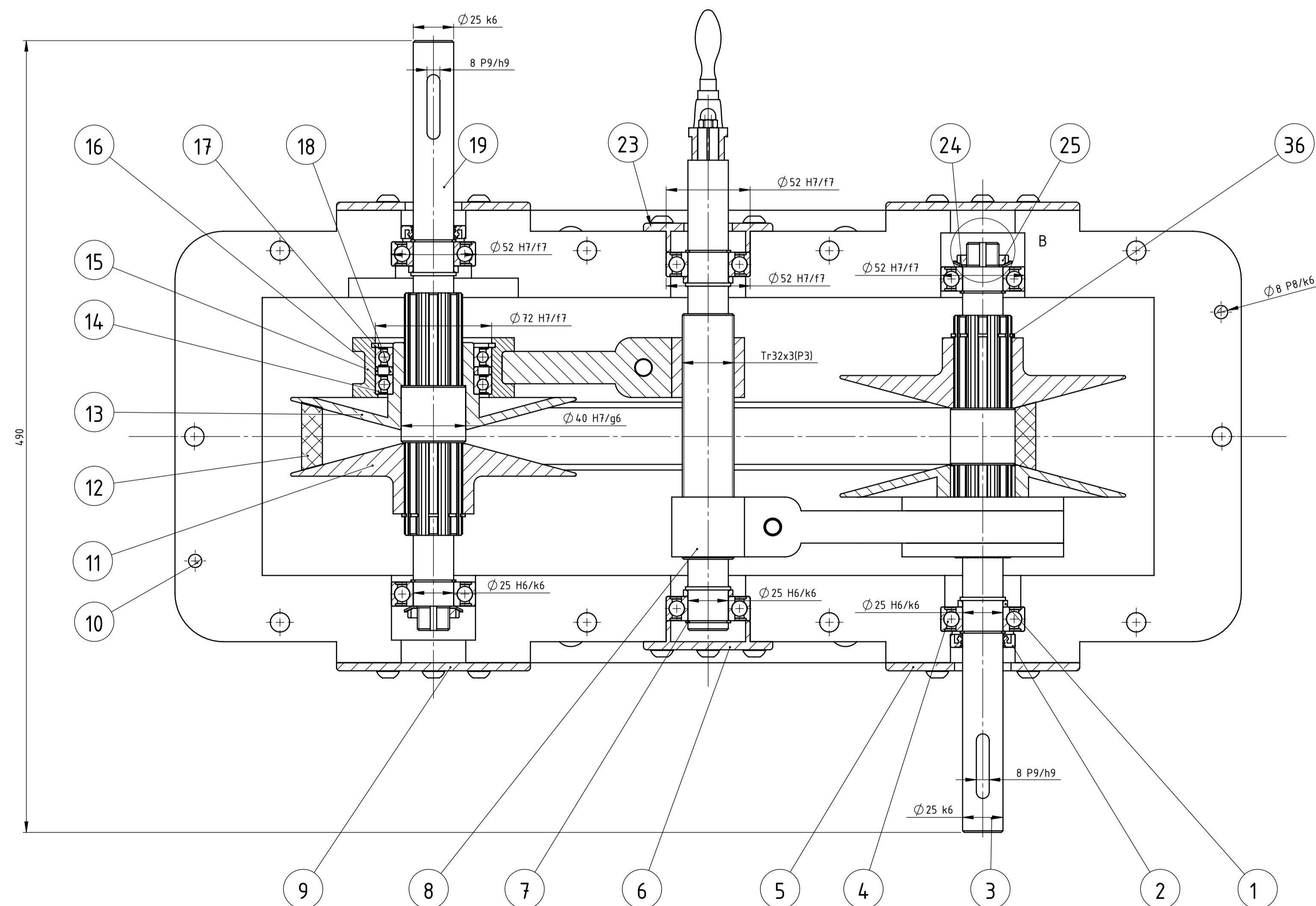
A-A (M 1:2)
