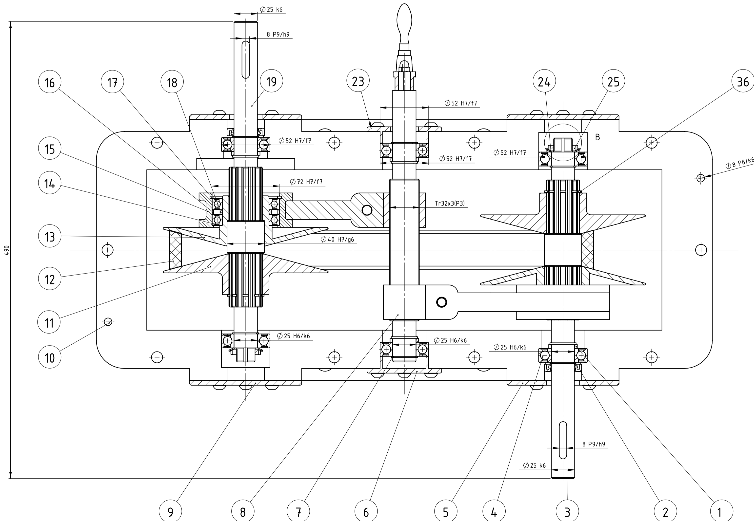
A-A (M 1:2)
