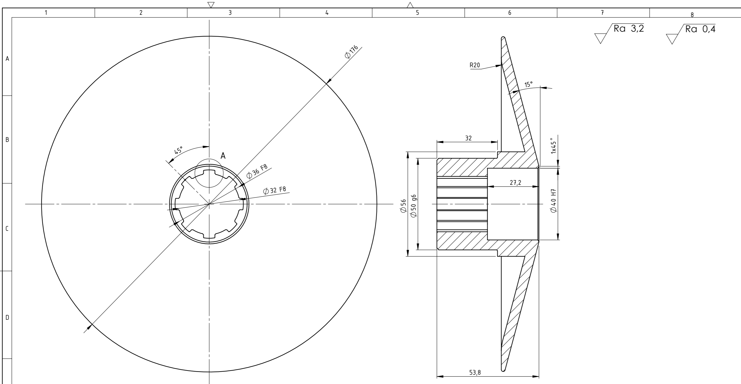
A (M 5 : 1)
