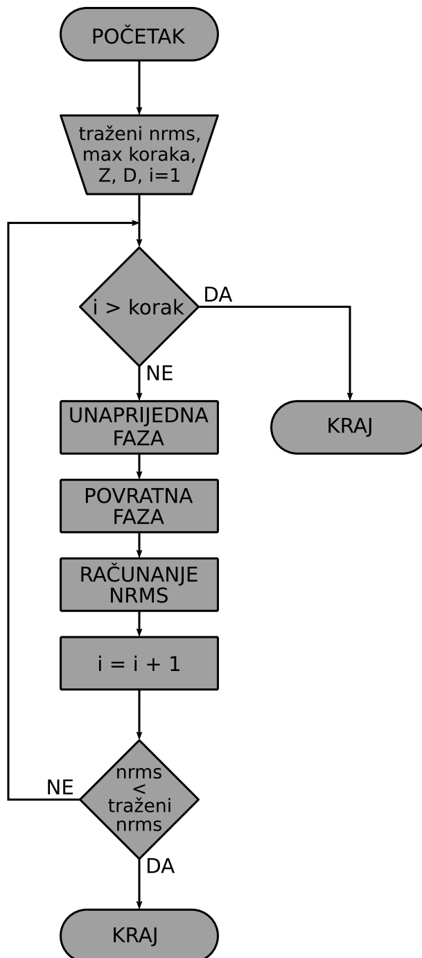
Slika 3.1: Dijagram toka algoritma učenja
