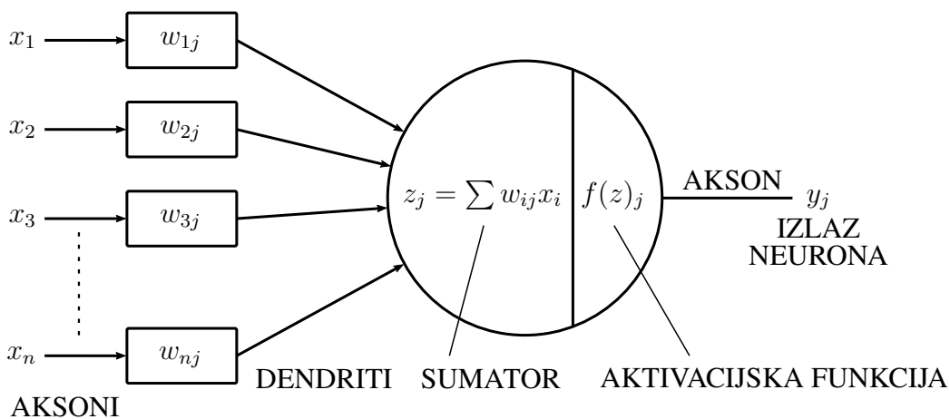
Slika 1.2: Struktura umjetnog neurona
