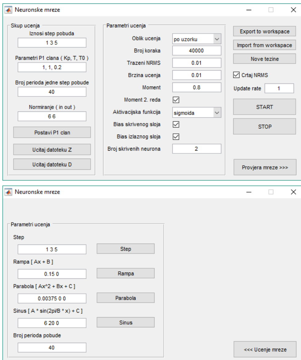
Slika 3.2: Grafičko sučelje
