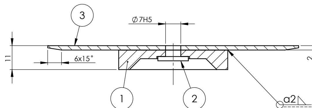
- Provrt se radi nakon zavarivanja diska (3) i graničnika (1) postupkom MIG zavarivanja. - Svornjak (2) se nalazi u dosjedu s vratilom s crteža IS-1000-1-07 te se zajedno sklapaju.
