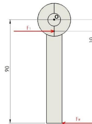
Slika 6: Sile na polugi
