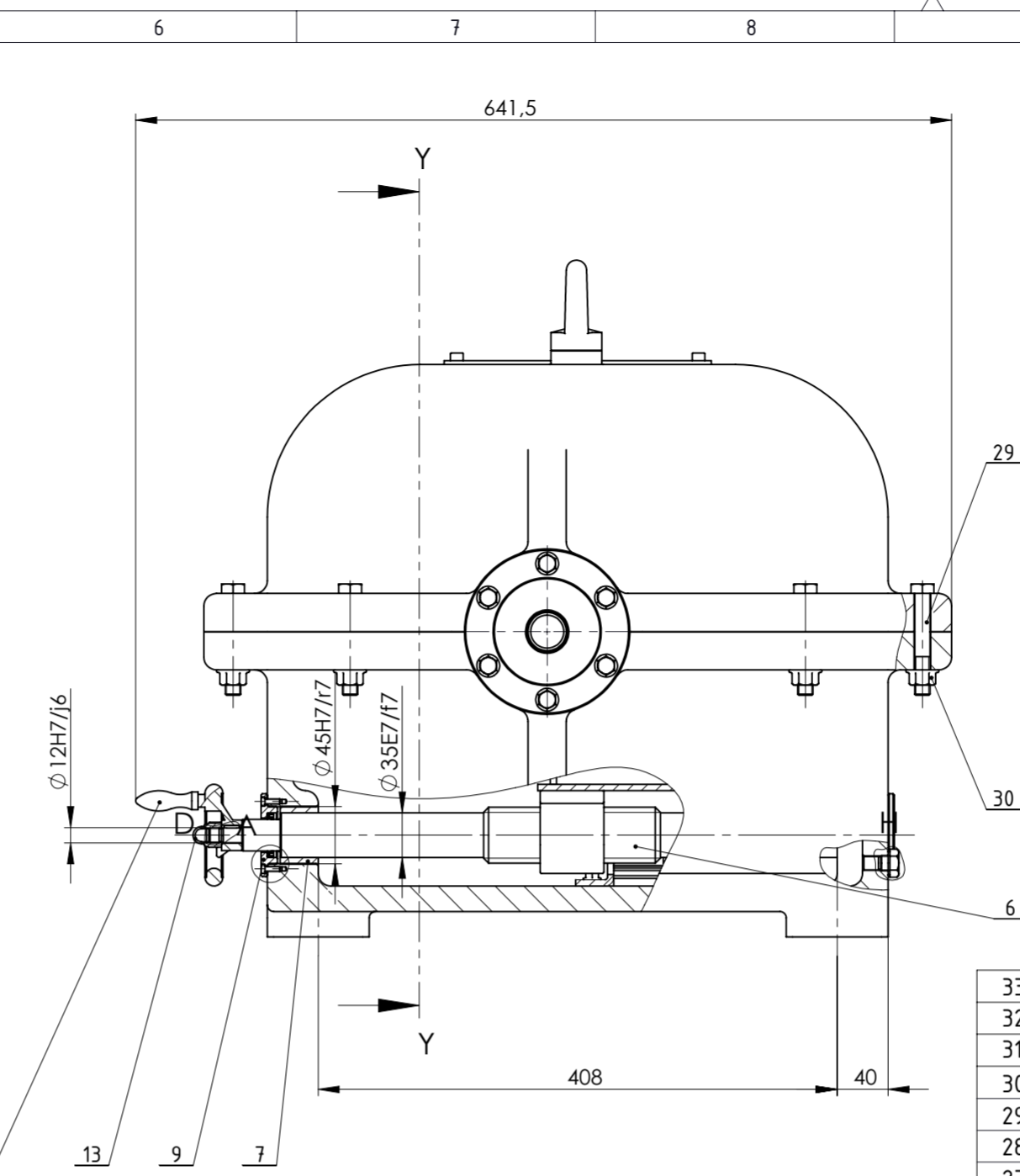
Presjek Y-Y
