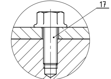
Detailj G M1:1
