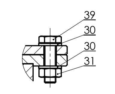
DETALJ J MJERILO 1 : 2
