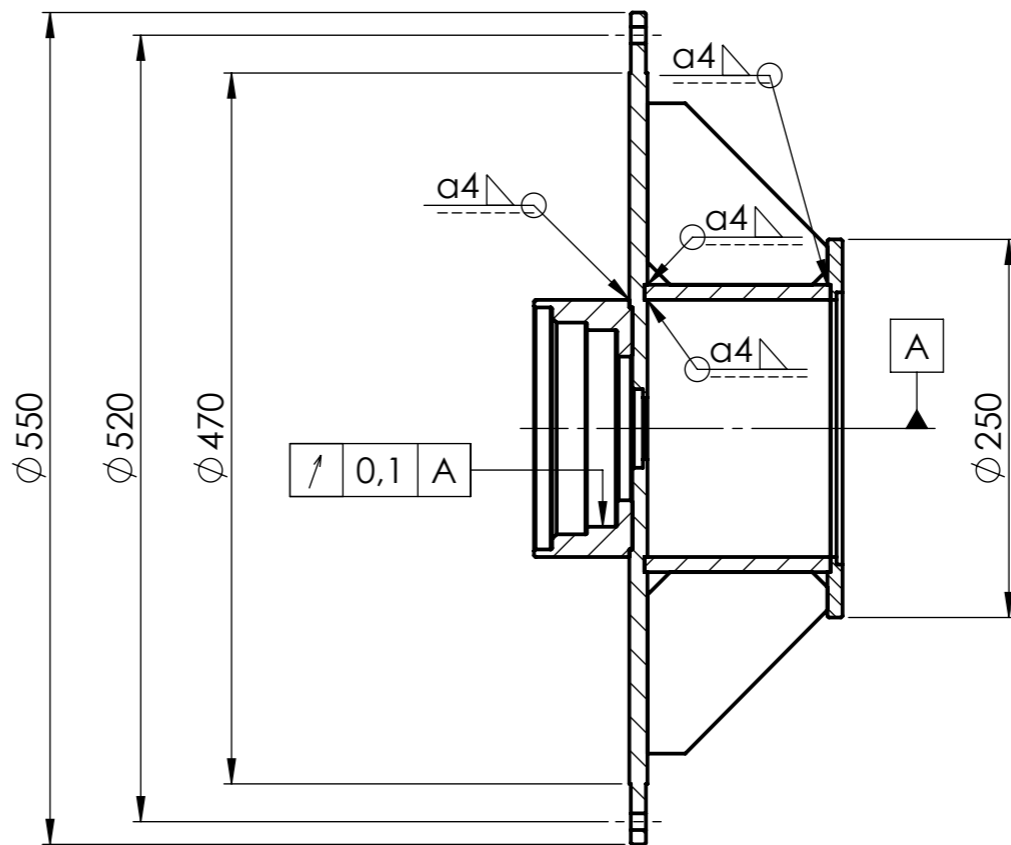
PRESJEK A-A
