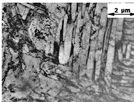
Slika 12 – Čelik bainitne mikrostrukture
