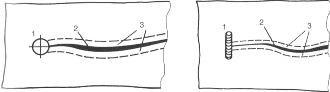
Slika 24. Način pripreme spoja za zavarivanje sivog lijeva na hladno [2]
