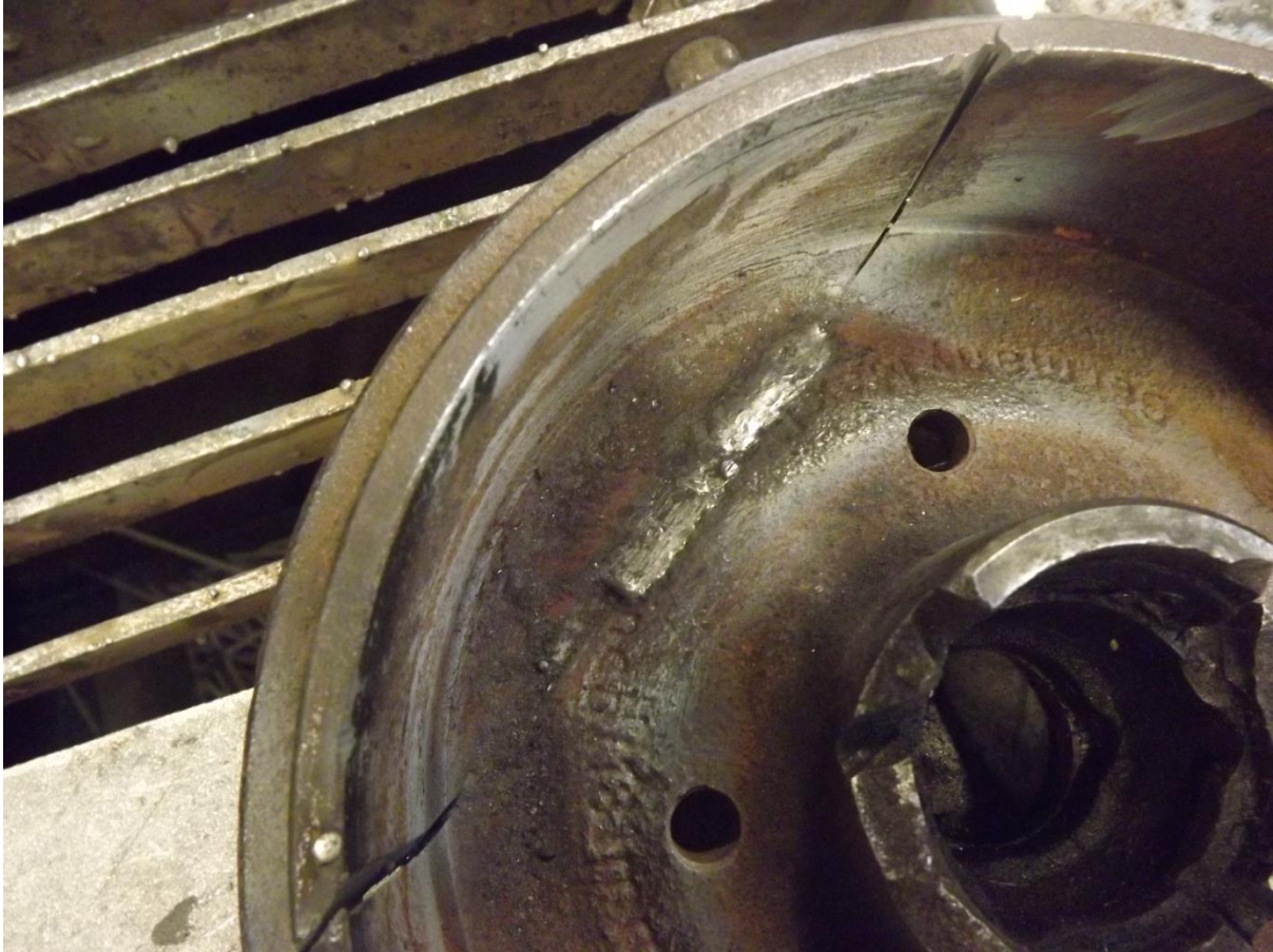
Slika 44. Korijen zavara
