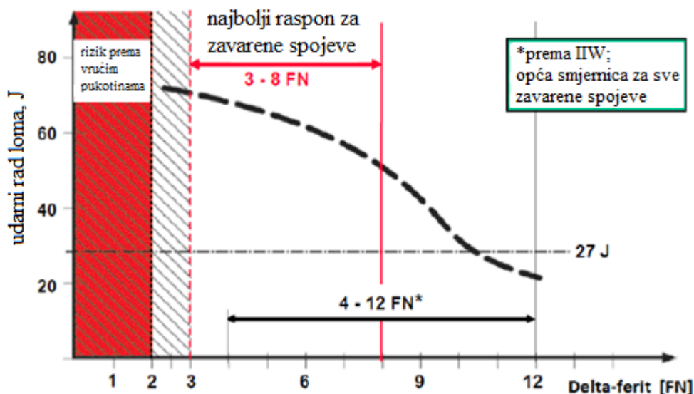
Slika 28. Utjecaj delta-ferita na iznos udarnog rada loma u metalu zavara pri -196 °C [37]
