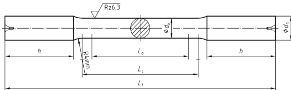
Slika 6.41. Dimenzije epruvete
