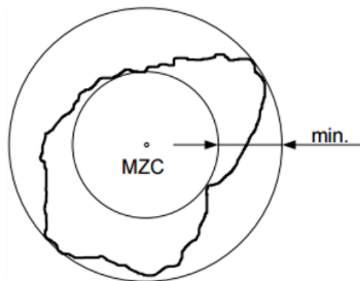
Slika 26. Chebysheva metoda [23]
