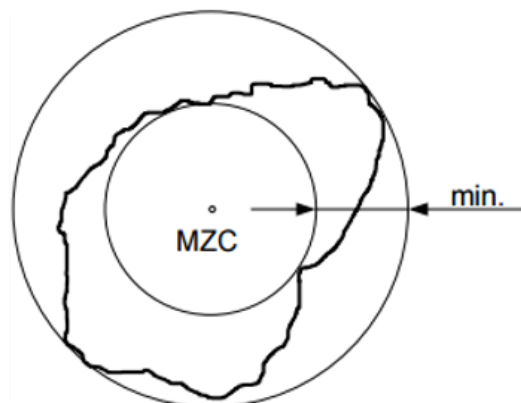
Slika 26. Chebysheva metoda [23]
