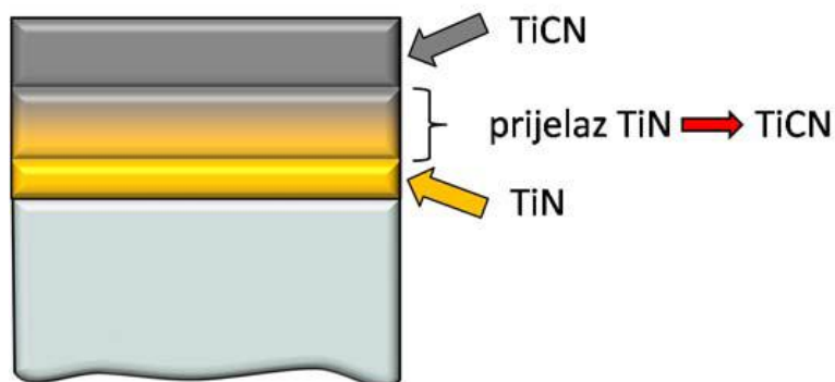
Slika 12. Shematski prikaz strukture gradijentne TiCN prevlake [9]
