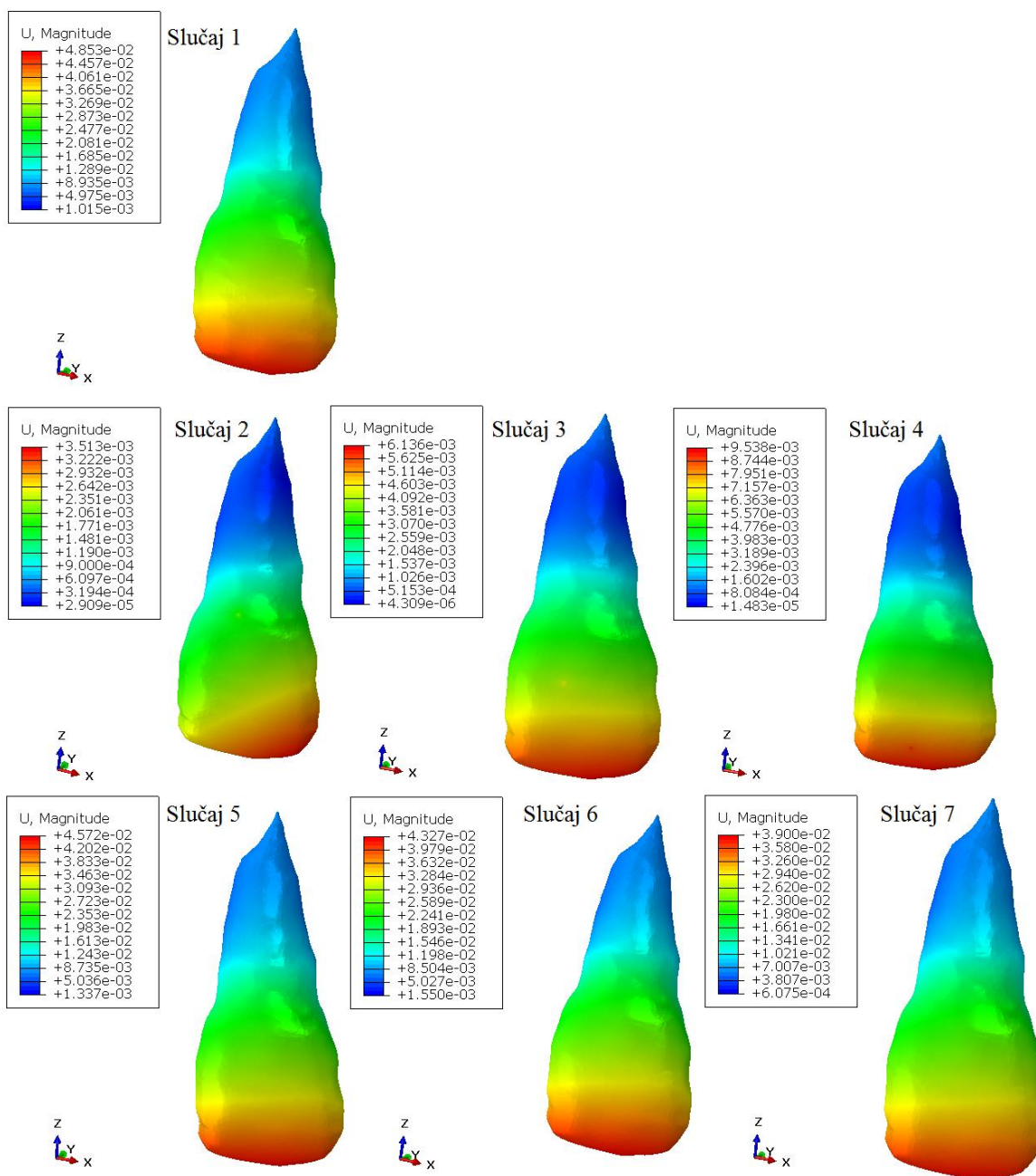
Slika 46. Prikaz pomaka zuba za svih sedam slučajeva opterećenja
