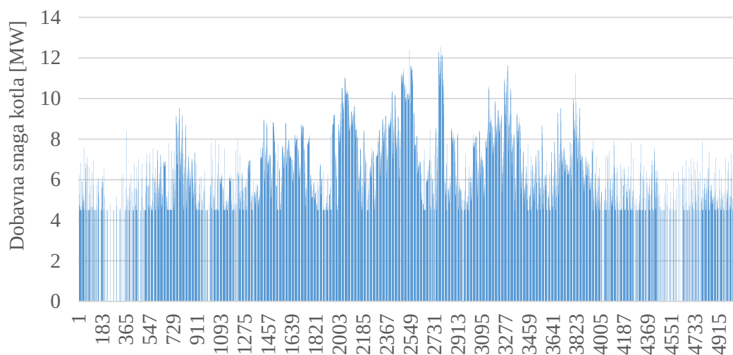
Slika 28. Satna raspodjela kotla na biomasu, distribucijska verzija 1, Scenarij 1
