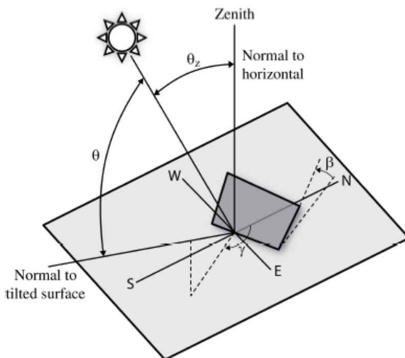
Slika 16. Pojašnjenje kutova vezanih za izračun direktnog zračenja na plohu pod određenim nagibom [42]
