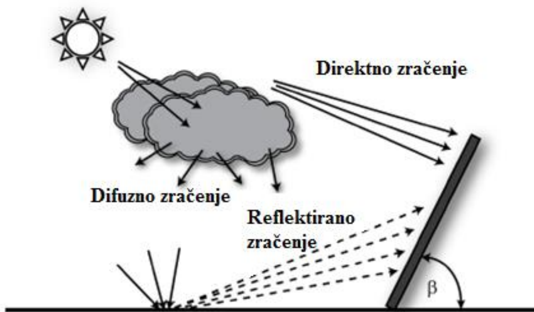
Slika 15. Ilustracija direktnog, difuznog i reflektiranog zračenja [42]
