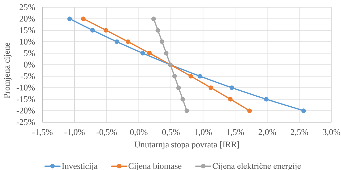
Slika 48. Analiza osjetljivosti, Scenarij 3, Kombinacija 1
