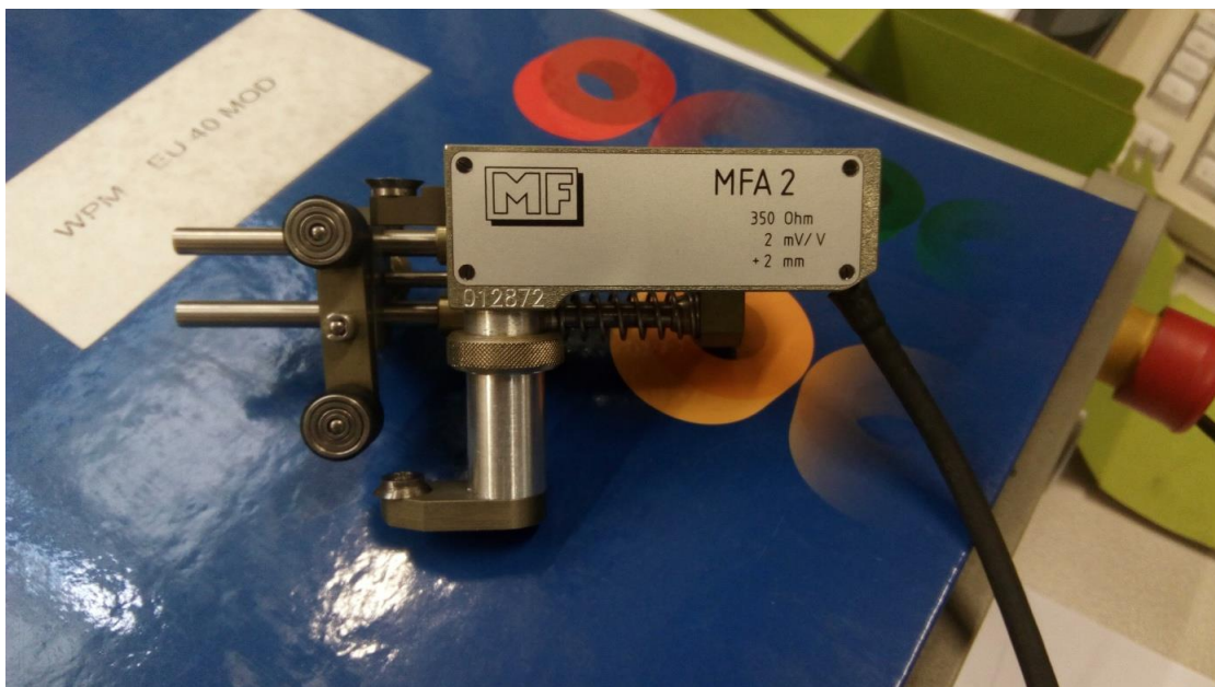
Slika 16. Ekstenzometar MFA 2
