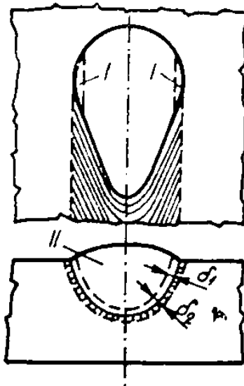
Slika 8. Prikaz zone taline metala zavara [15]
