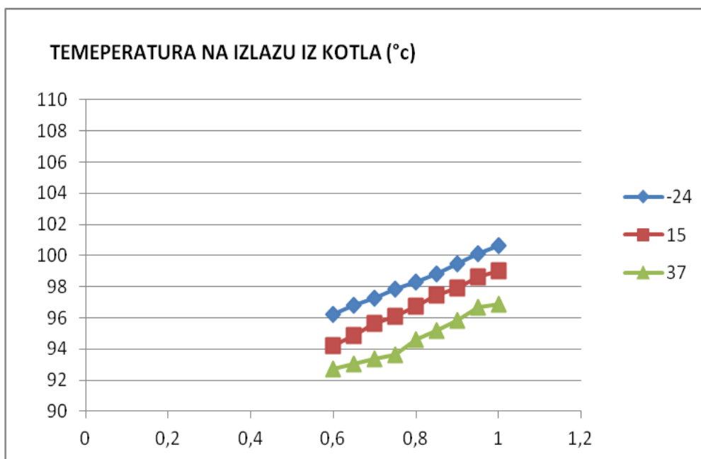
Slika 35. Temperatura na izlazu iz kotla T_{gi}(9) ( ^{\circ}\text{C} ) (0MW)
