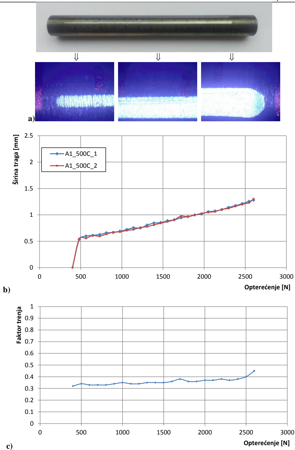
Slika 35. Rezultati trošenja ispitnog uzorka A1_500C: a) Izgled istrošene površine, b) ovisnost širine traga trošenja o opterećenju, c) ovisnost faktora trenja o opterećenju
