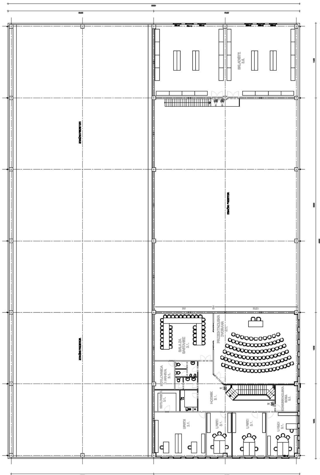
Slika 2.6. Tlocrt kata hale III [3]
