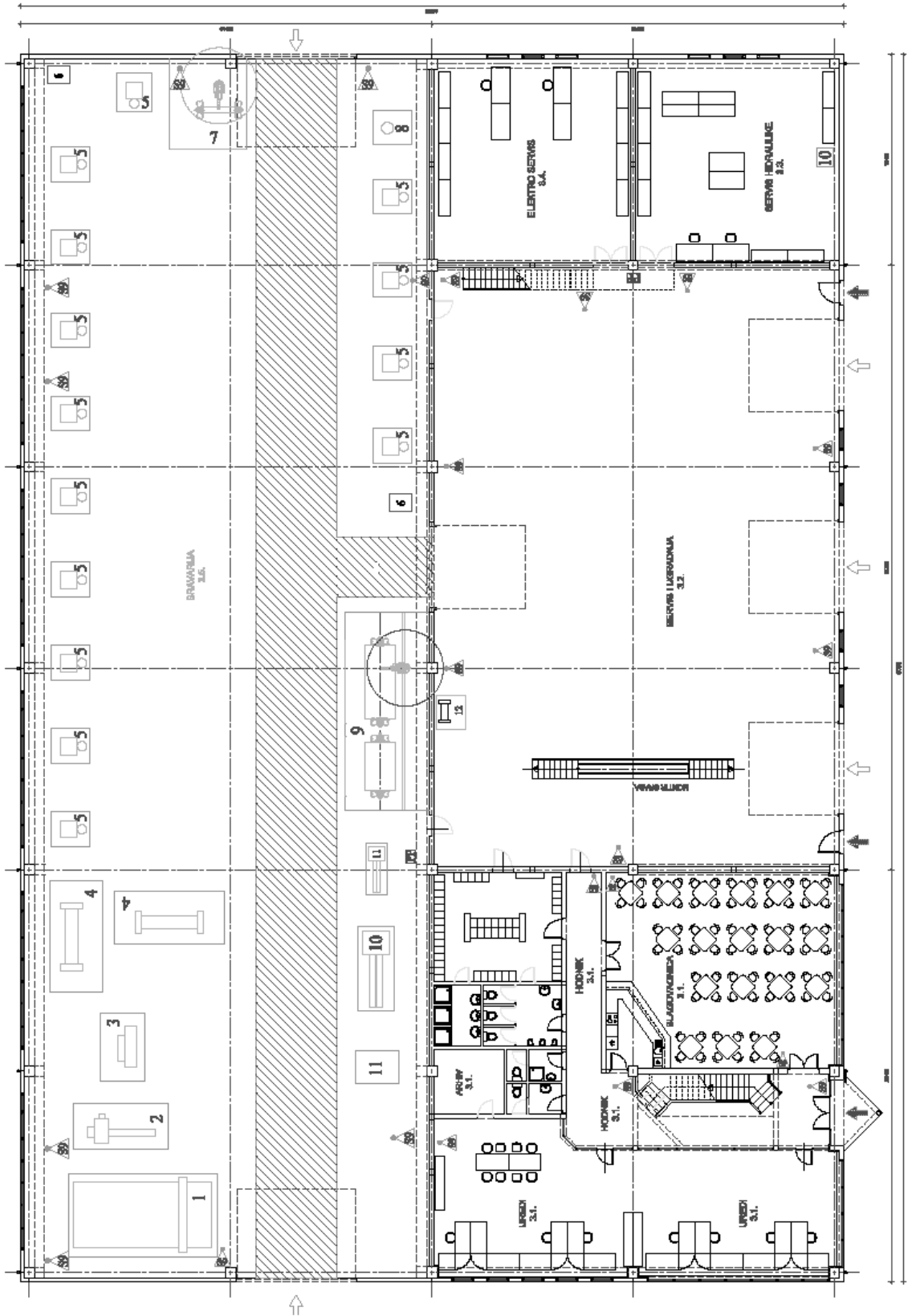
Slika 2.5. Tlocrt prizemlja hale III [3]
