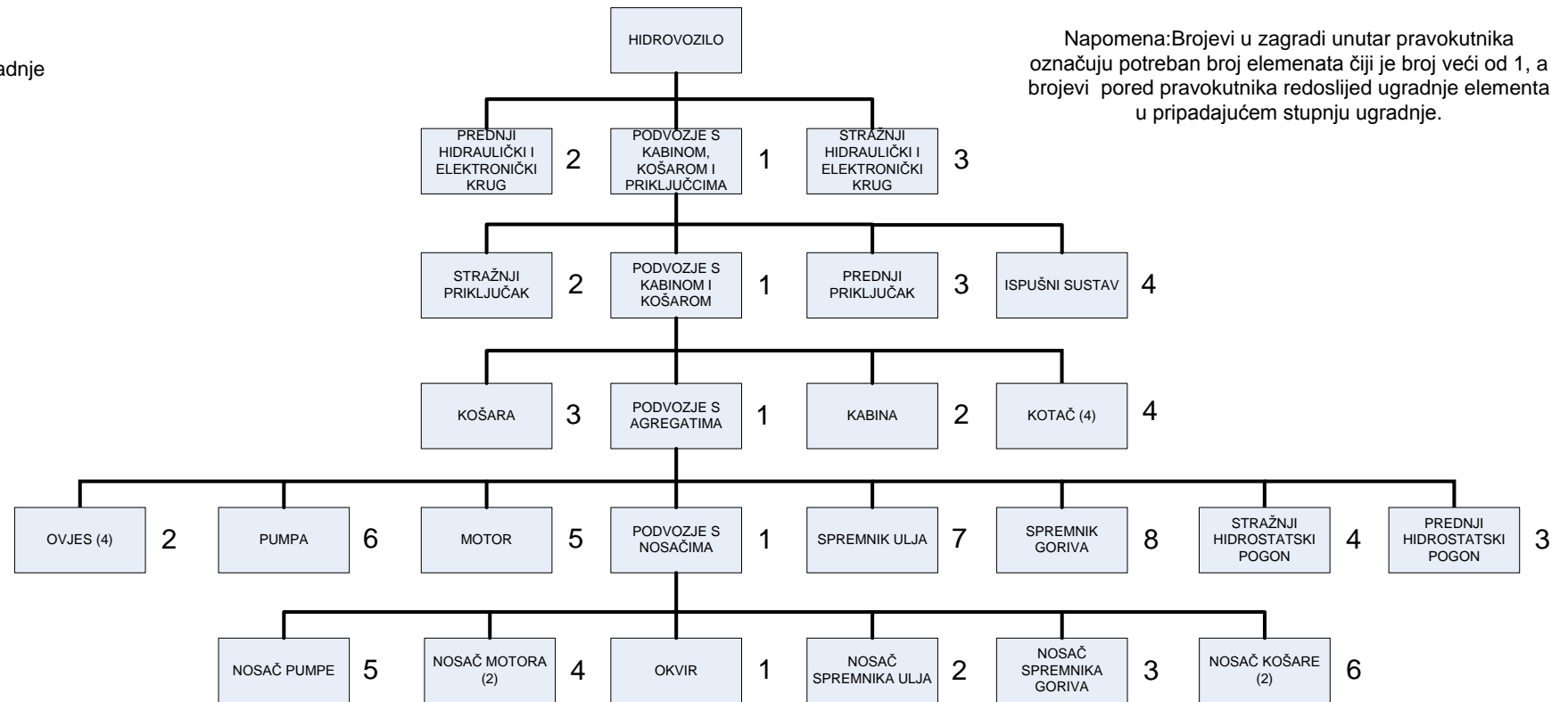
Slika 4.3. Redoslijed sklapanja
