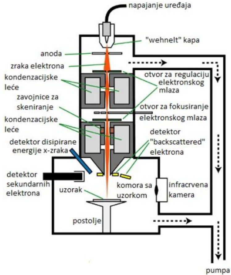
Slika 29. Shema skenirajućeg elektronskog mikroskopa
