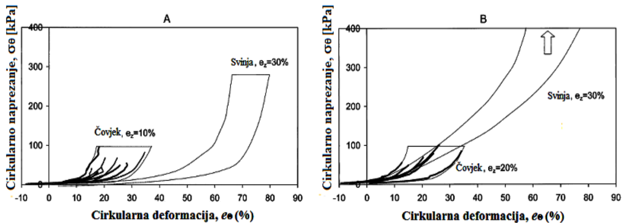
Slika 6. Usporedba odnosa cirkularnog naprezanja u ovisnosti o cirkularnoj deformaciji za ljudske i svinjske arterije [29]
