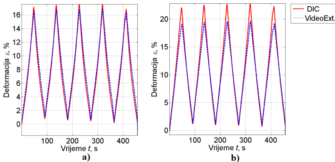
Slika 107. Usporedni prikaz promjene deformacije \varepsilon u vremenu t za Prekondicioniranje 2 uzorka AORTA 3 u a) aksijalnom (A) i b) transverzalnom (T) smjeru za DIC i videoekstenzometar
