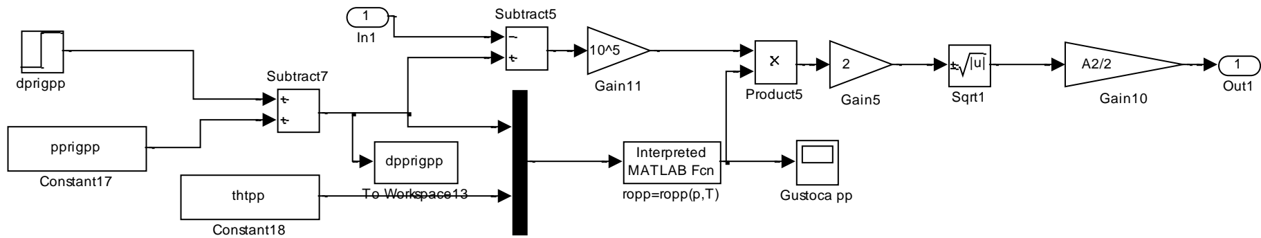
Shema Simulink modela jednačbe strujanja pregrijane pare
