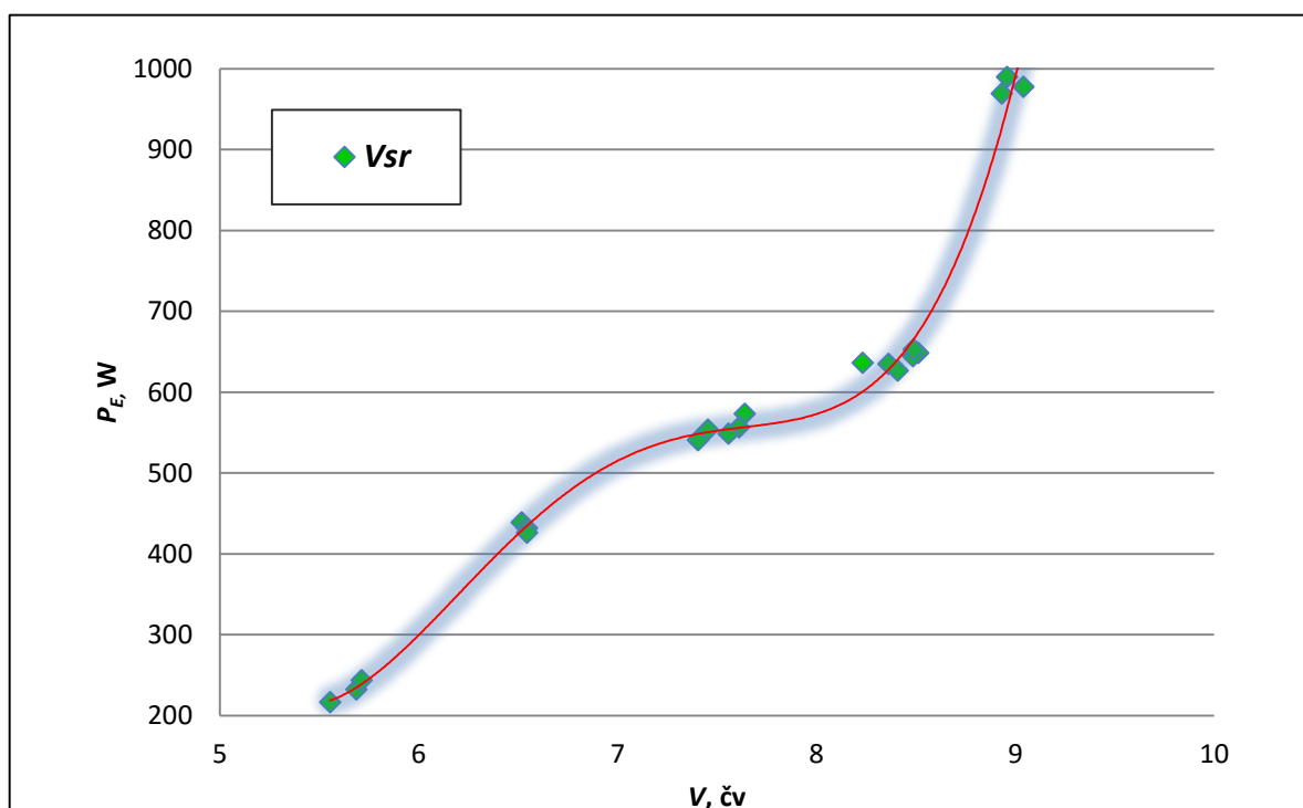
Slika 41. Ovisnost snage i srednje vrijednosti brzine brodocikla u trećoj vožnji
