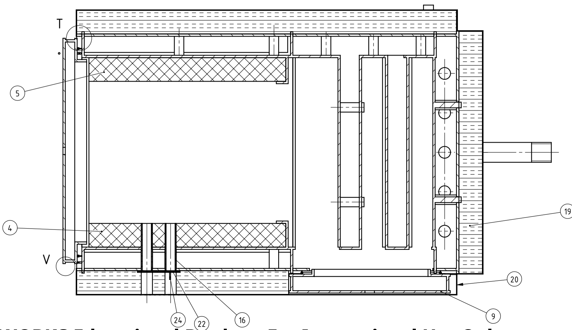
PRESJEK B-B
