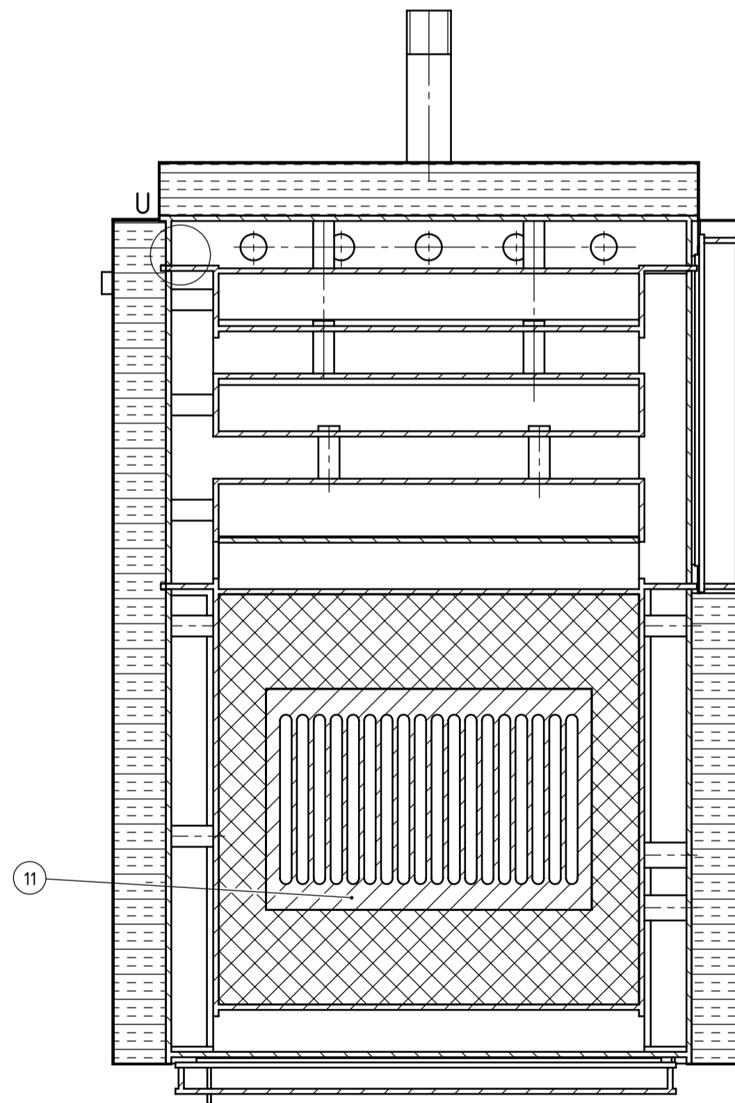
PRESJEK C-C
