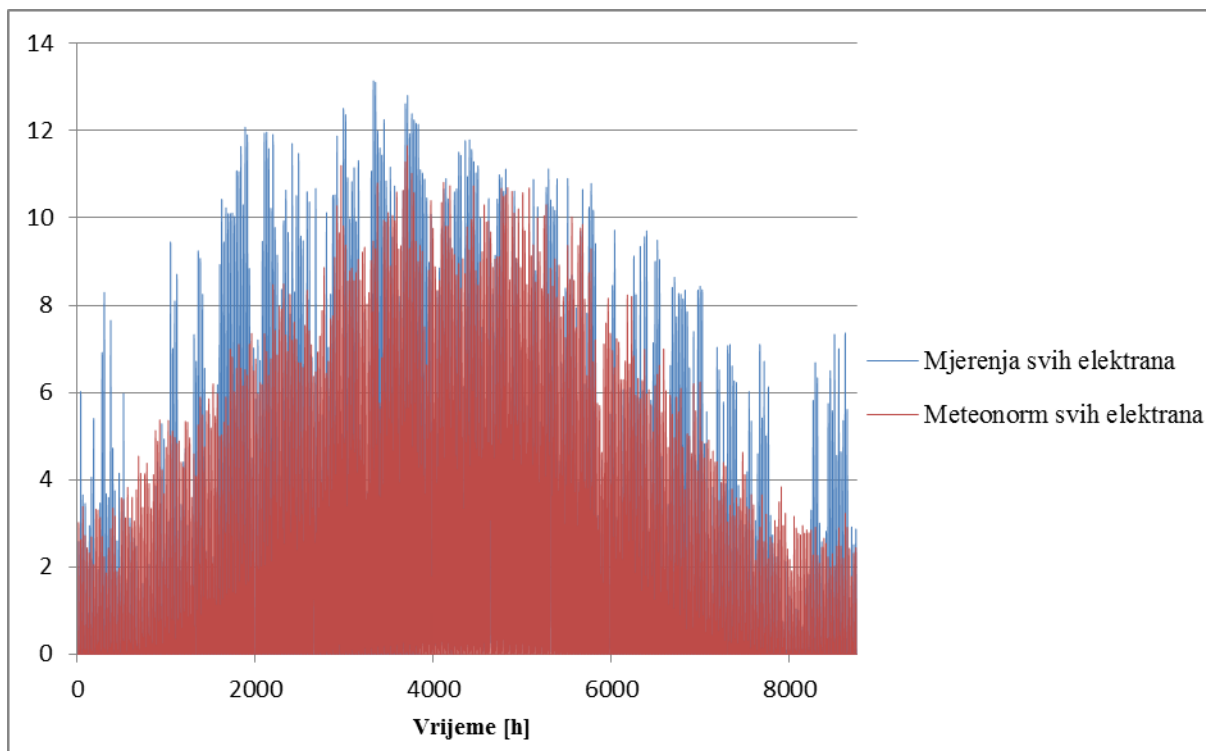
Slika 20. Prikaz usporedbe podataka o relativnoj proizvodnji električne energije iz mjerenih izvora i podataka o relativnoj dozračenju energiji iz baza Meteoronorma u bezdimenzijskom obliku
