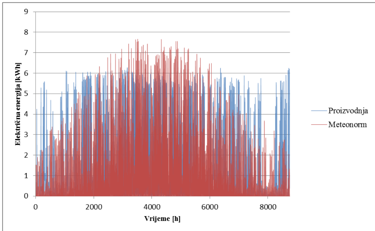
Slika 18. Usporedba podataka o proizvodnji električne energije iz mjerenih izvora i Meteonorma za sunčanu elektranu Solarni stup Špansko
