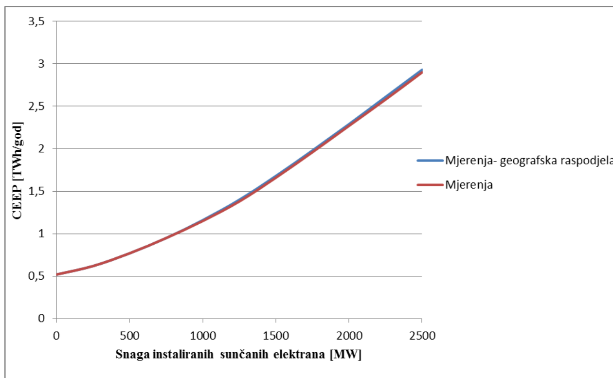
Slika 26. Rast CEEP-a u ovisnosti o kapacitetima instaliranih sunčanih elektrana i geografskoj lokaciji elektrana za usporedbu podataka o proizvedenoj električnoj energiji preuzetih sa Sunnyportala
