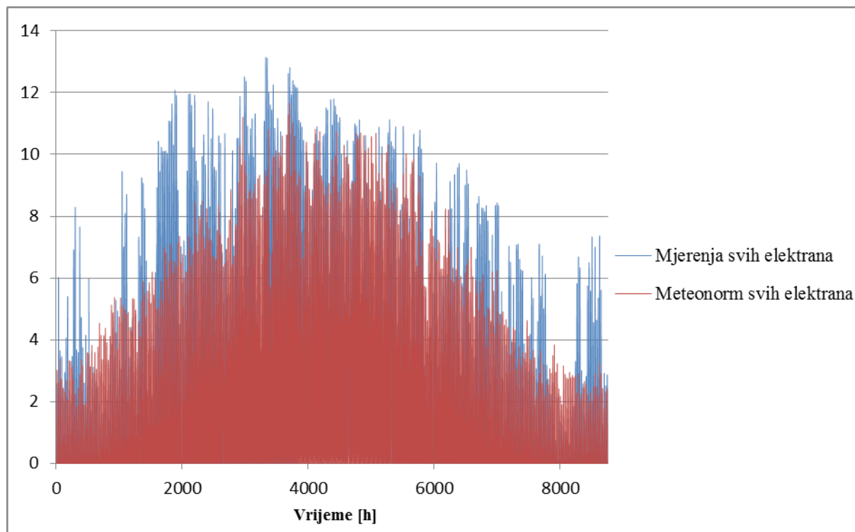
Slika 20. Prikaz usporedbe podataka o relativnoj proizvodnji električne energije iz mjerenih izvora i podataka o relativnoj dozračenoj energiji iz baza Meteororma u bezdimenzijskom obliku
