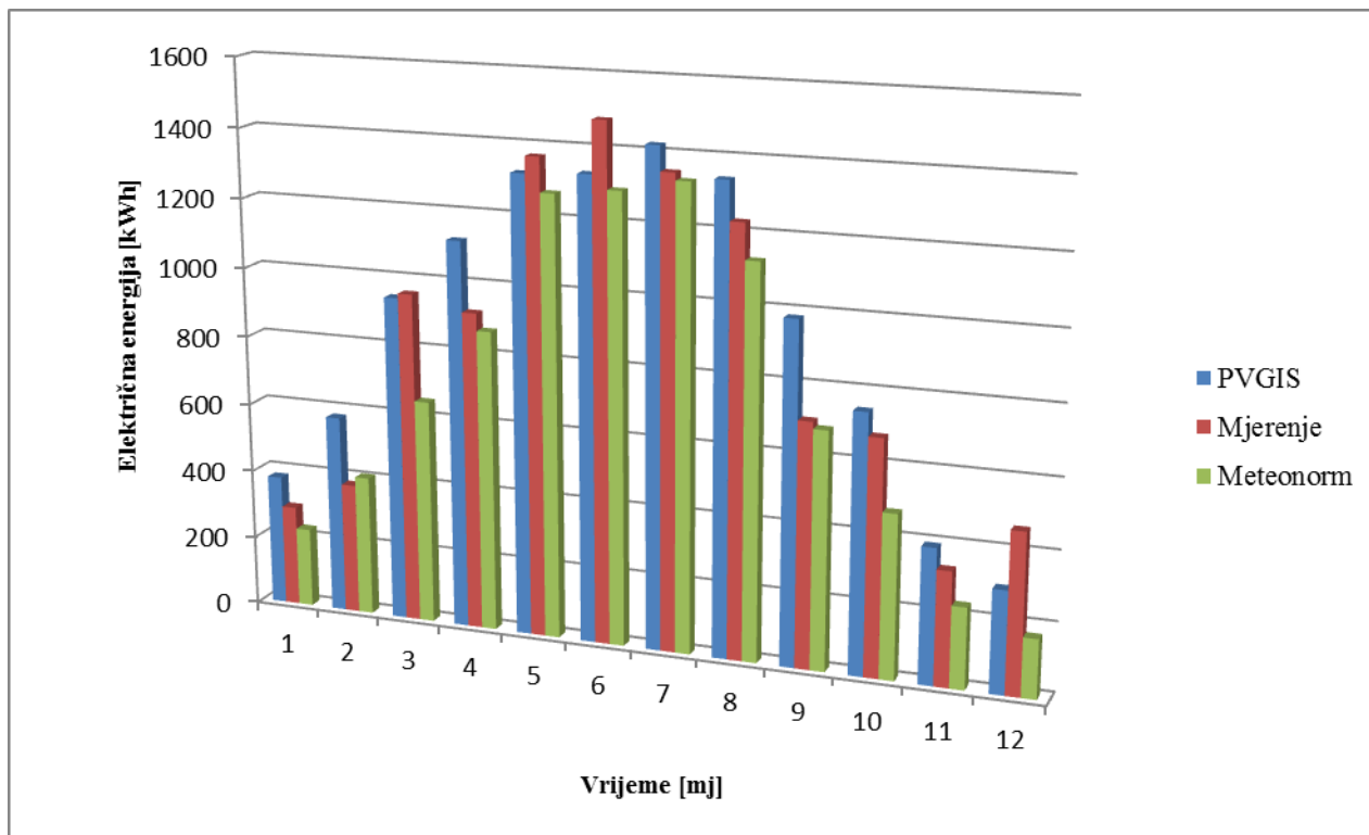
Slika 19. Mjesečna usporedba proizvodnje električne energije iz mjerenih podataka, Meteoroma i PVGIS-a sunčane elektrane Solarni stup Špansko
