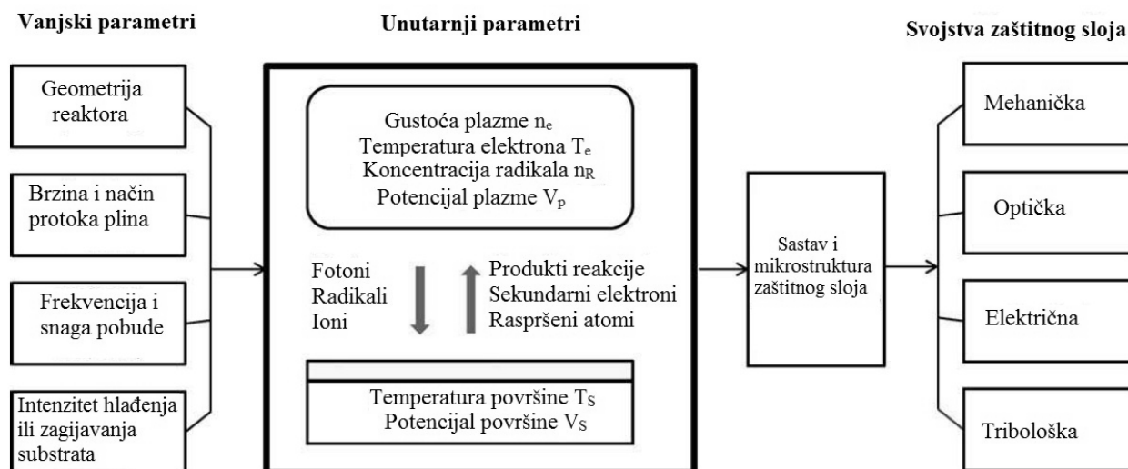
Slika 2.2 Shematski prikaz veze između vanjskih i unutrašnjih parametara sa svojstvima PACVD sloja [5]
