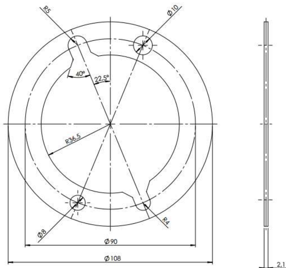
Slika 19. Brtva – nacrt.
