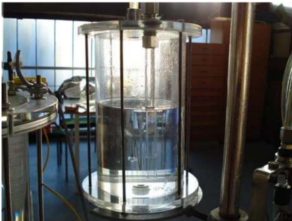
Slika 33. Spremnik elektrolita [2].
