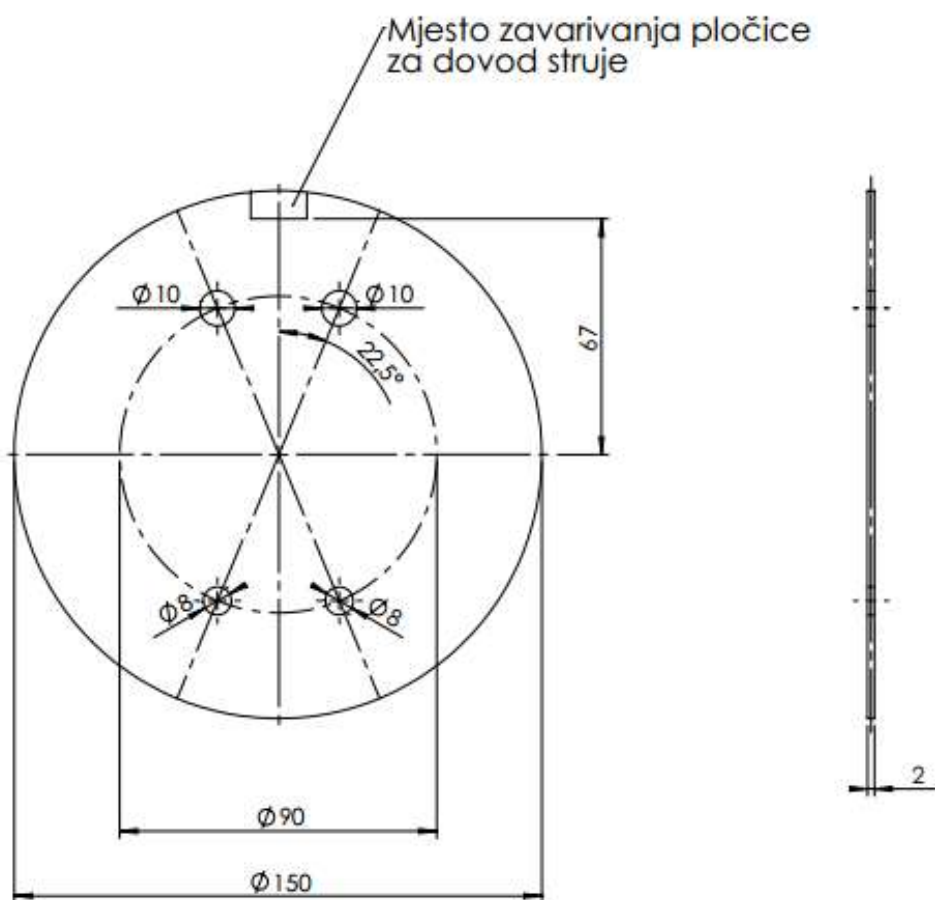
Slika 13. Monopolarna ploča – nacrt.
