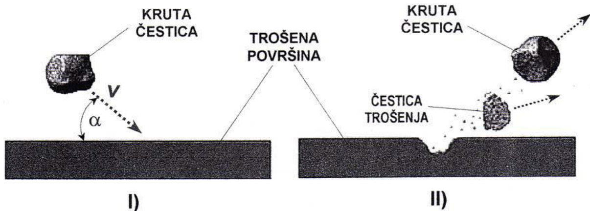
Slika 14. Jedinični događaj procesa erozije česticama [5]
