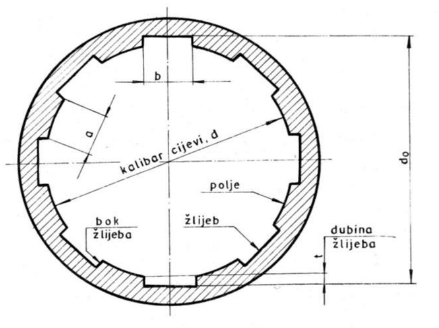
Slika 3. Poprečni presjek cijevi [1]
