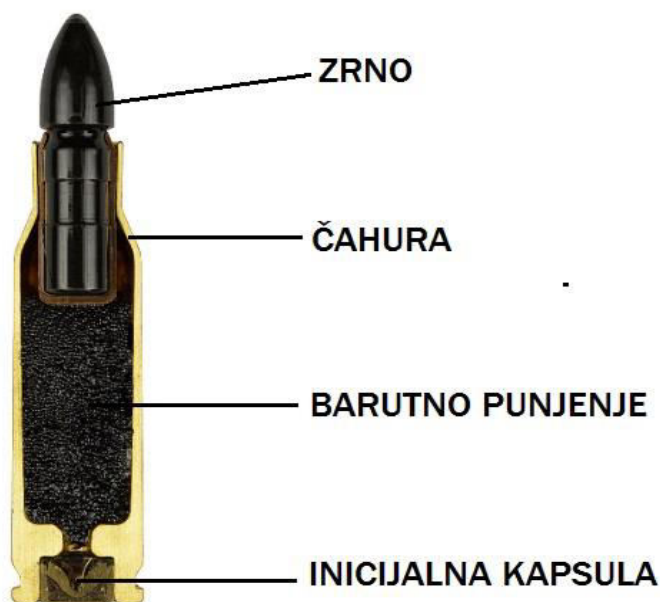
Slika 7. Poprečni presjek metka [8]
