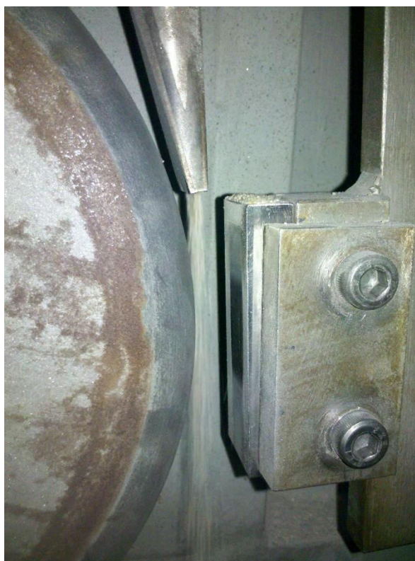
Slika 21. Detalj uređaja i trag trošenja na uzorku
