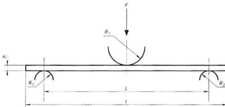
Slika 25. Shema ispitivanja savojne čvrstoće [23]
