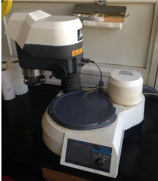
Slika 28 Uređaj za strojno brušenje metalografskih uzoraka
