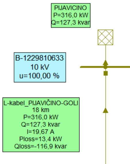
Slika 50. Tok snage prema Pelješcu sa zapada
