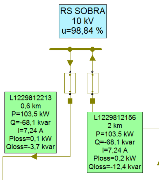
Slika 47. Sabirnica
